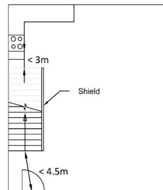
(d) Open plan arrangement for escape - shield to stairs
